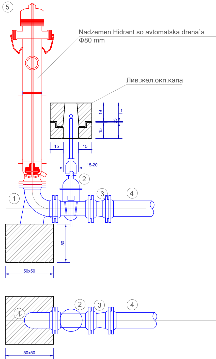
Детал на надземен ПП хидрант со приклучок на ПП мрежа
