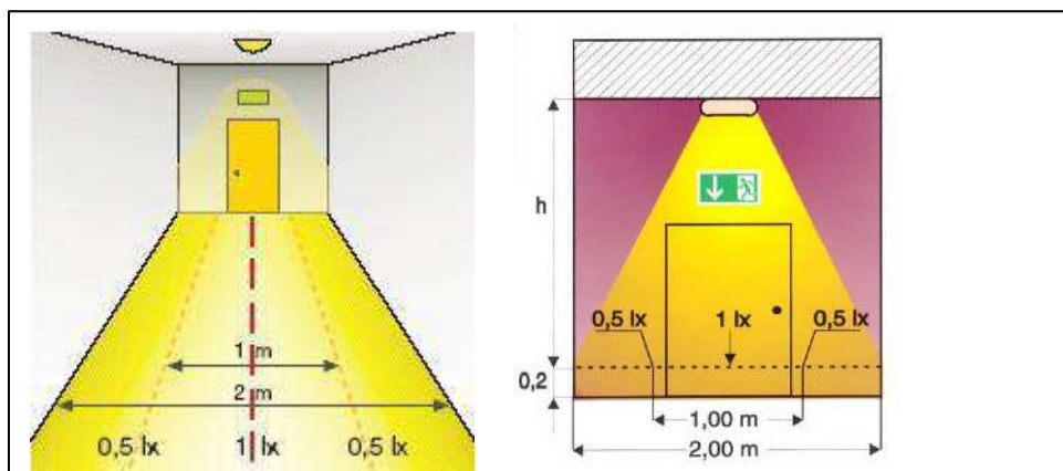
(Слика 6.1) Потребна ширина на коридорот за евакуација
