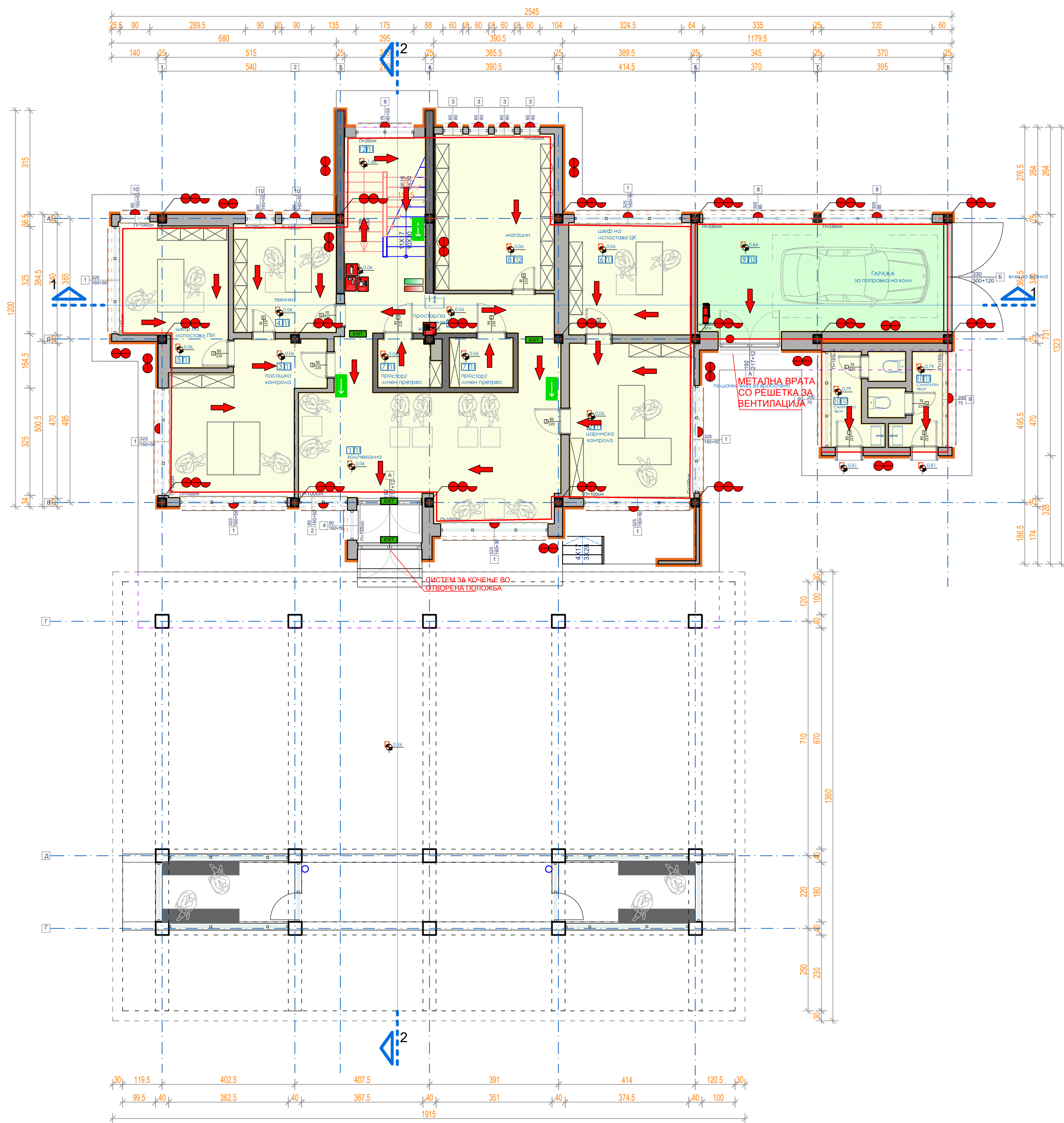
ОСНОВА НА ПРИЗЕМЈЕ СО МЕБЕЛ (НИВО -0.06)
