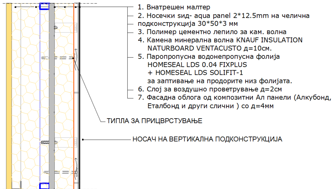
(Слика 3.3.3.1) Новопроектиран монтажен сид
